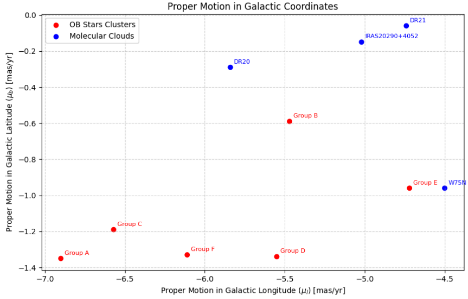
FIGURE 12 – Mouvement propre selon la latitude galactique \mu_b en fonction du mouvement propre selon la longitude galactique \mu_l , les nuages moléculaires sont en bleus et les amas d'étoiles OB en rouge
