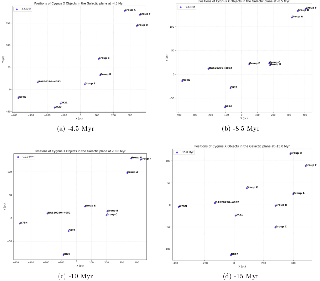
FIGURE 10 – Traceback linéaire sur le plan galactique des objets du Cygne à -4.5, -8.5, -10 et -15 Myr.
